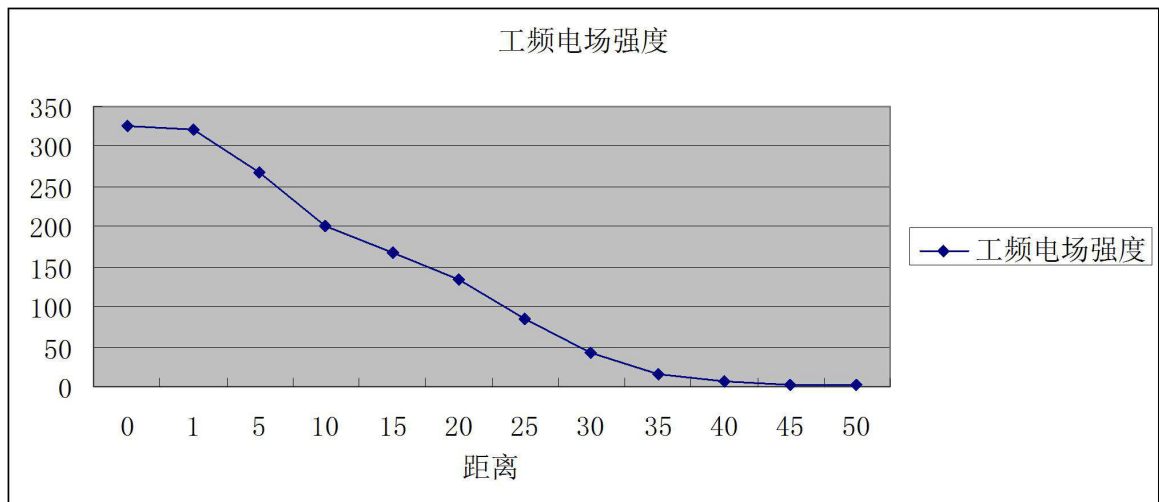
图 3-7 类比单回架空线路工频电场强度分布趋势图
