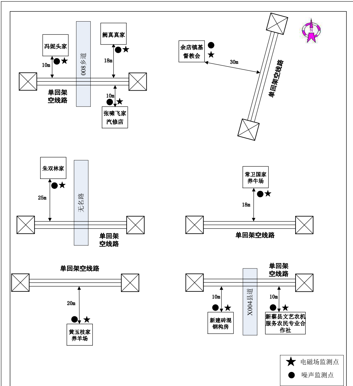
图5 110kV 输变电线线路敏感点监测布点图
