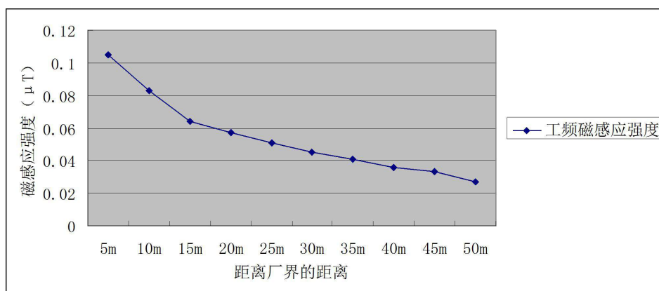
图 3-3 类比电站磁感应强度变化图
