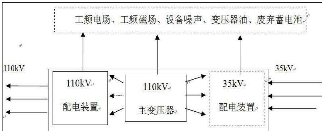
图 7 升压站运行期工艺流程及产污环节图
