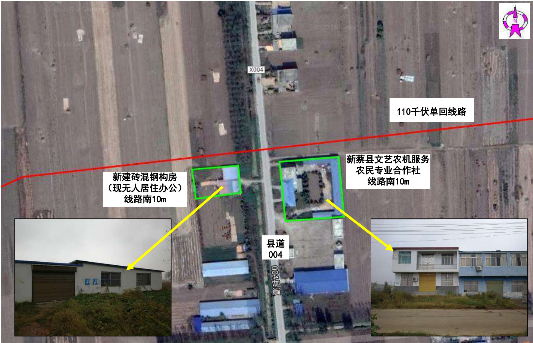
图3-6 陈店镇敏感目标与工程位置关系图及现场图片（6）
