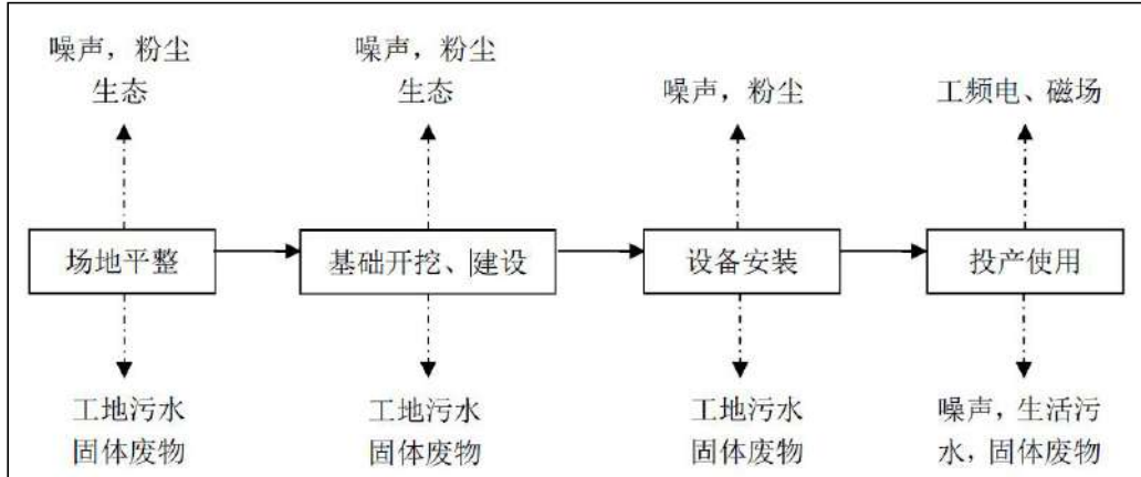
图 6 升压站施工期工艺流程及产污环节图
