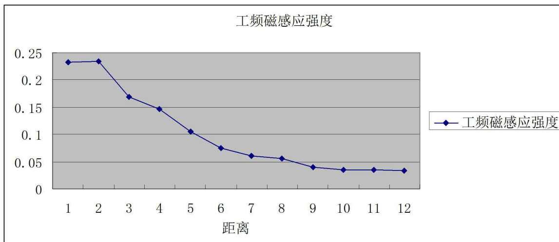
图 3-8 类比单回架空线路磁感应强度分布趋势图
