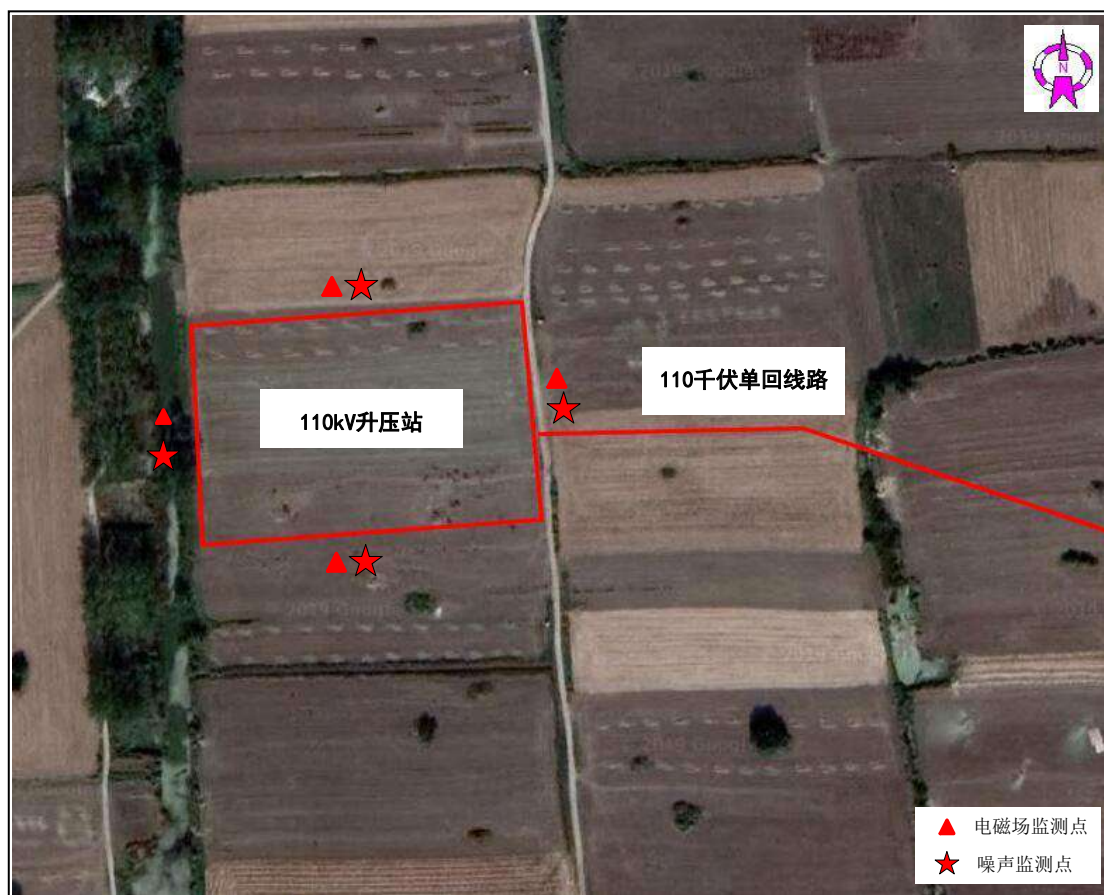
图4 风电场 110kV 升压站监测布点图
