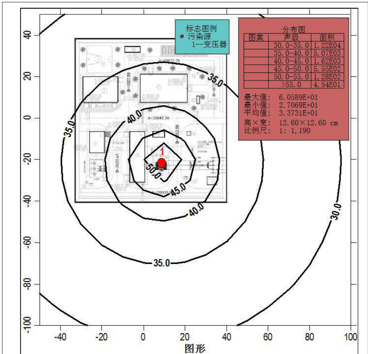
图 9 项目噪声预测等声级线图
