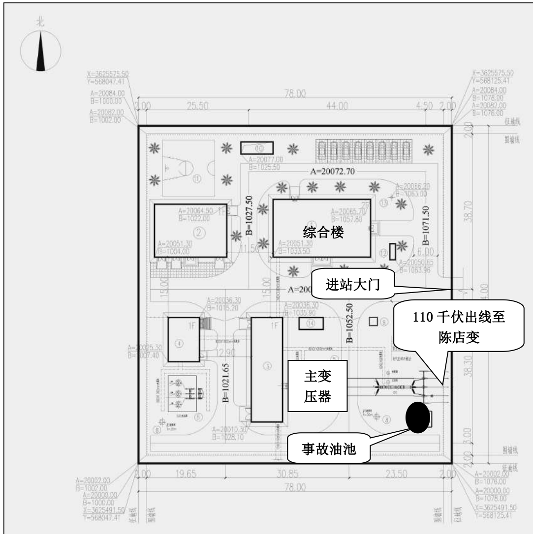
图 1 升压站平面布置图
